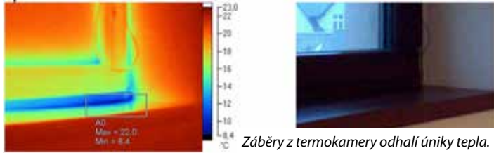
Záběry z termokamery odhalí úniky tepla.
